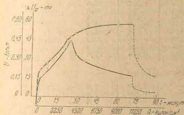
Рис. 3. Зависимость потенциала и фотогальванического эффекта Au-электрода в 1 N H_2SO_4 от поляризации (свет белый) \circ - \circ - \circ — потенциал электрода; \times - \times - \times — фотогальванический эффект (Q в микрокулонах)
