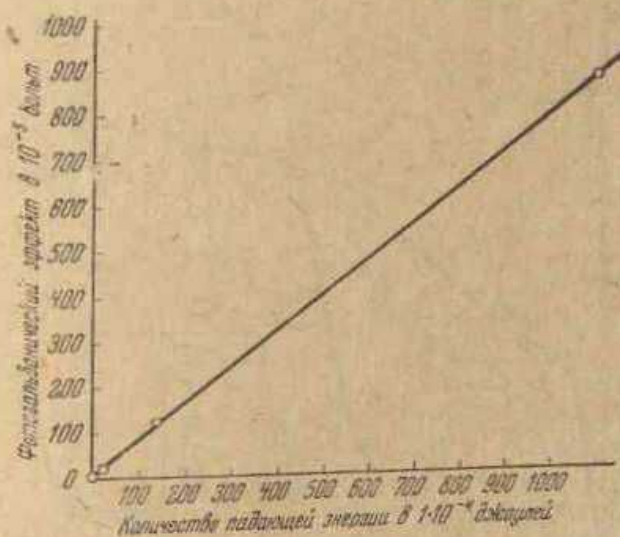
Рис. 8. Зависимость величины фотогальванического эффекта от интенсивности излучения
