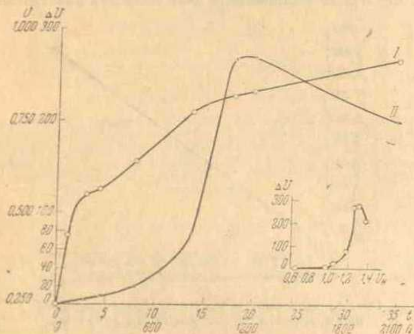
Рис. 9. Зависимость потенциала фотогальванического эффекта Au-электрода в 1N \text{ KNO}_3 от поляризации: кривая I — потенциал электрода; кривая II — фотогальванический эффект ( Q в микрокулонах)
