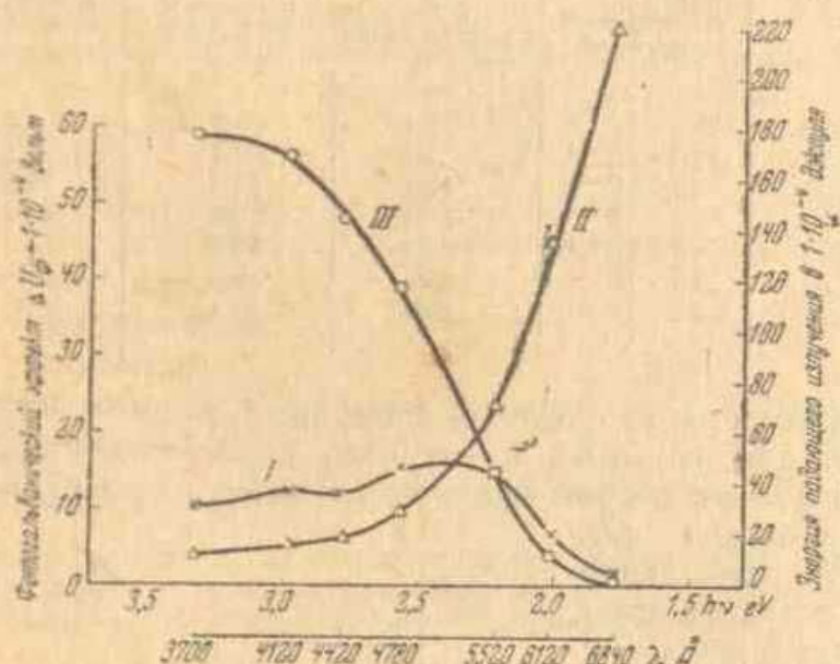
Рис. 7. Спектральная чувствительность фотогальванического эффекта Au-электрода в 1 \text{ N H}_2\text{SO}_4 : кривая I — экспериментальные значения фотогальванического эффекта; кривая II — количества падающей энергии; кривая III — величины фотогальванического эффекта, приведенные к равным энергиям
