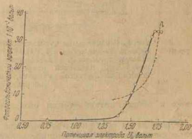
Рис. 6. Зависимость фотогальванического эффекта Au-электрода от потенциала: о — о — о — первая поляризация; х — х — х — повторная поляризация
