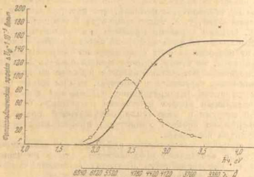
Рис. 12. Зависимость спектральной чувствительности фотогальванического эффекта Au-электрода от энергии падающего кванта излучения: X—X—X—значения фотогальванического эффекта, приведенные к равному количеству квант; o—o—o—относительный прирост величины фотогальванического эффекта
