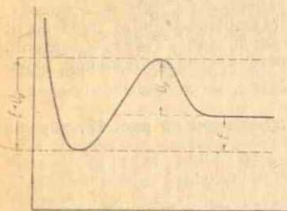
Рис. 13. E — энергия связи адсорбированного фотогальванического комплекса; U_V — высота потенциального барьера процесса; E + U_V — энергия элементарного фотогальванического акта
