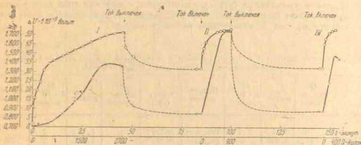
Рис. 5. Зависимость потенциала и фотогальванического эффекта Au-электрода от количества пропущенного электричества при повторных поляризациях. \circ-\circ-\circ- потенциал электрода; \times-\times-\times- фотогальванический эффект ( Q в микрокулонах)
