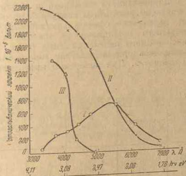
Рис. 10. Спектральная чувствительность фотогальванического эффекта Au-электрода в 1 \text{ N KNO}_3 : кривая I — экспериментальные значения фотогальванического эффекта; кривая II — величины фотогальванического эффекта, приведенные к равным энергиям; кривая III — спектральная чувствительность Au-электрода по данным Кларка и Гаррета.
