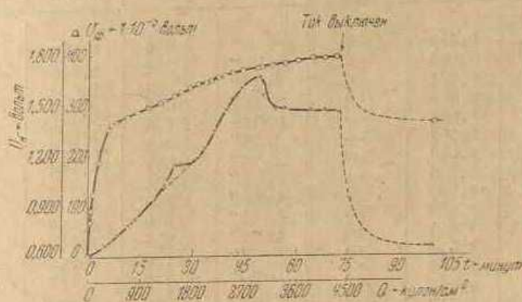
Рис. 4. Зависимость потенциала и фотогальванического эффекта Au-электрода в 1 N H_2SO_4 от поляризации (свет монохроматический). \circ - \circ - \circ — потенциал электрода; \times - \times - \times — фотогальванический эффект (Q в микрокулонах)
