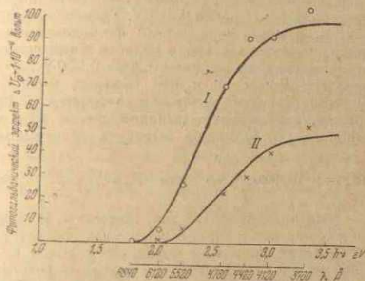
Рис. 11. Зависимость спектральной чувствительности фотогальванического эффекта Au-электрода от потенциала: кривая I — V_n = 1,716 вольт; кривая II — V_n = 1,500 вольт
