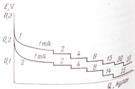
Рис. 2. Электровосстановление аллилового спирта. 1 — раствор 0,1N H_2SO_4 ; 2 — 0,1N NaOH
