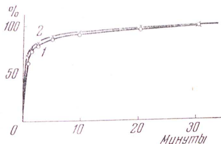
Рис. 3. Кинетика удаления водорода с электрода. 1 — раствор 0,1N \text{HS}_2\text{O}_4 ; 2 — 0,1N NaOH
