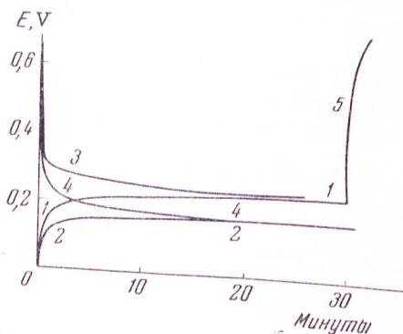
Рис. 1. Кривые 1, 3, 5 соответствуют раствору 0,1N H_2SO_4 ; 2, 4— 0,1N NaOH
