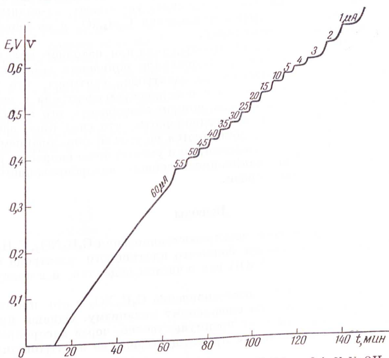
Рис. 3. Кривая электровосстановления C_6H_5NO_2 в 0,1 N NaOH
