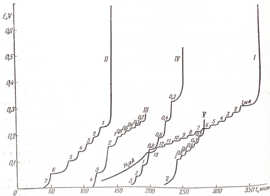
Рис. 1. Кривые электровосстановления пнробензола, фенилгидроксиламина и n -нитрофенола: I — C_6H_5NO_2 в 0,1 N H_2SO_4 ; II — C_6H_5NO_2 в 0,01 N HCl; III — C_6H_5NO_2 в 50% C_2H_5OH , подкисленном до 0,1 N H_2SO_4 ; IV — C_6H_5NHOH в 50% C_2H_5OH , подкисленном до 0,1 N H_2SO_4 ; V — C_6H_4(NO_2)(OH) в 50% C_2H_5OH , подкисленном до 0,1 N H_2SO_4 .
