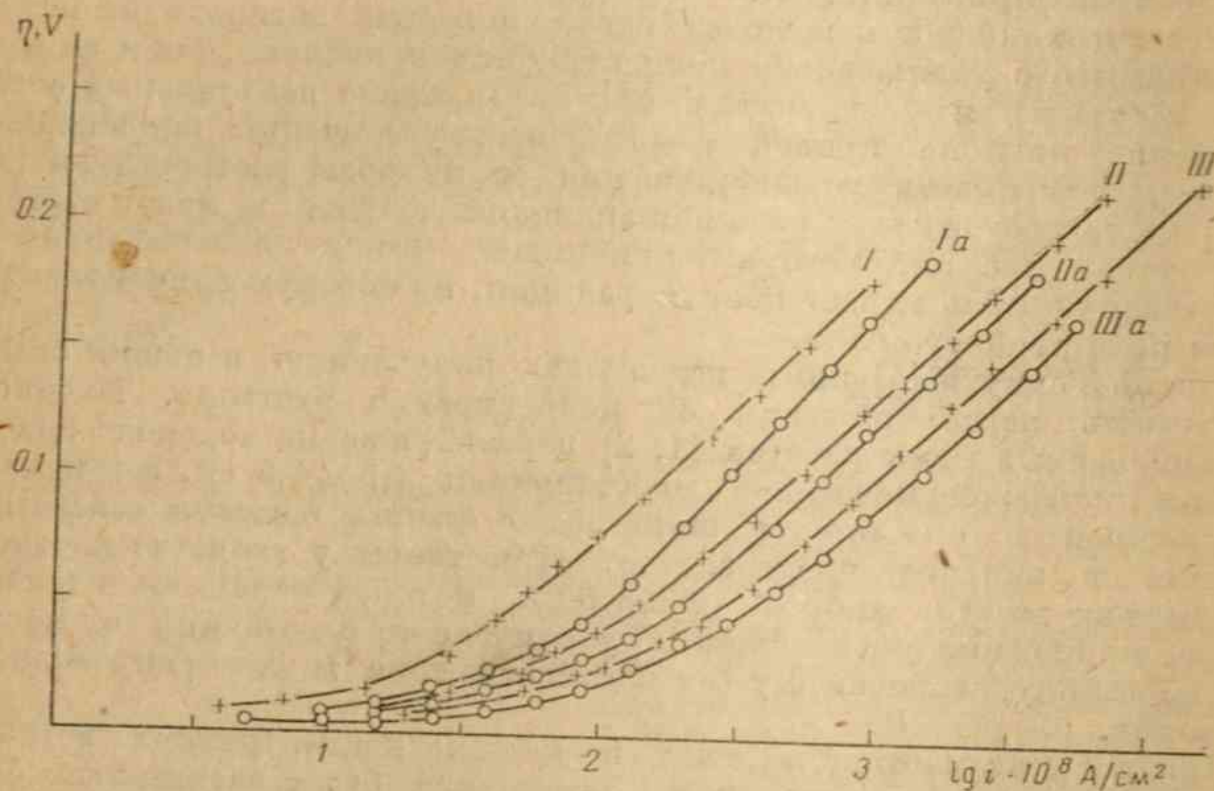
Рис. 1. Влияние формы электрода на перенапряжение в растворах щелочей различных концентраций: I — 0,83 \cdot 10^{-3} N NaOH; Ia — 3,9 \cdot 10^{-3} N NaOH; II — 4,10 \cdot 10^{-2} N NaOH; IIa — 0,9 \cdot 10^{-1} N NaOH; III — 2,80 \cdot 10^{-1} N NaOH; IIIa — 4,3 \cdot 10^{-1} N NaOH
