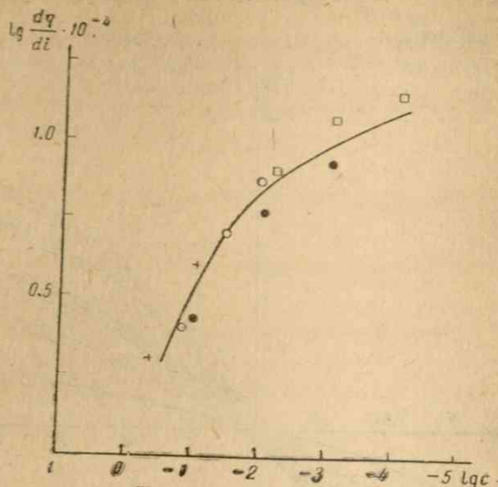
Рис. 6. Зависимость „сопротивления“ электрода от концентрации NaOH
