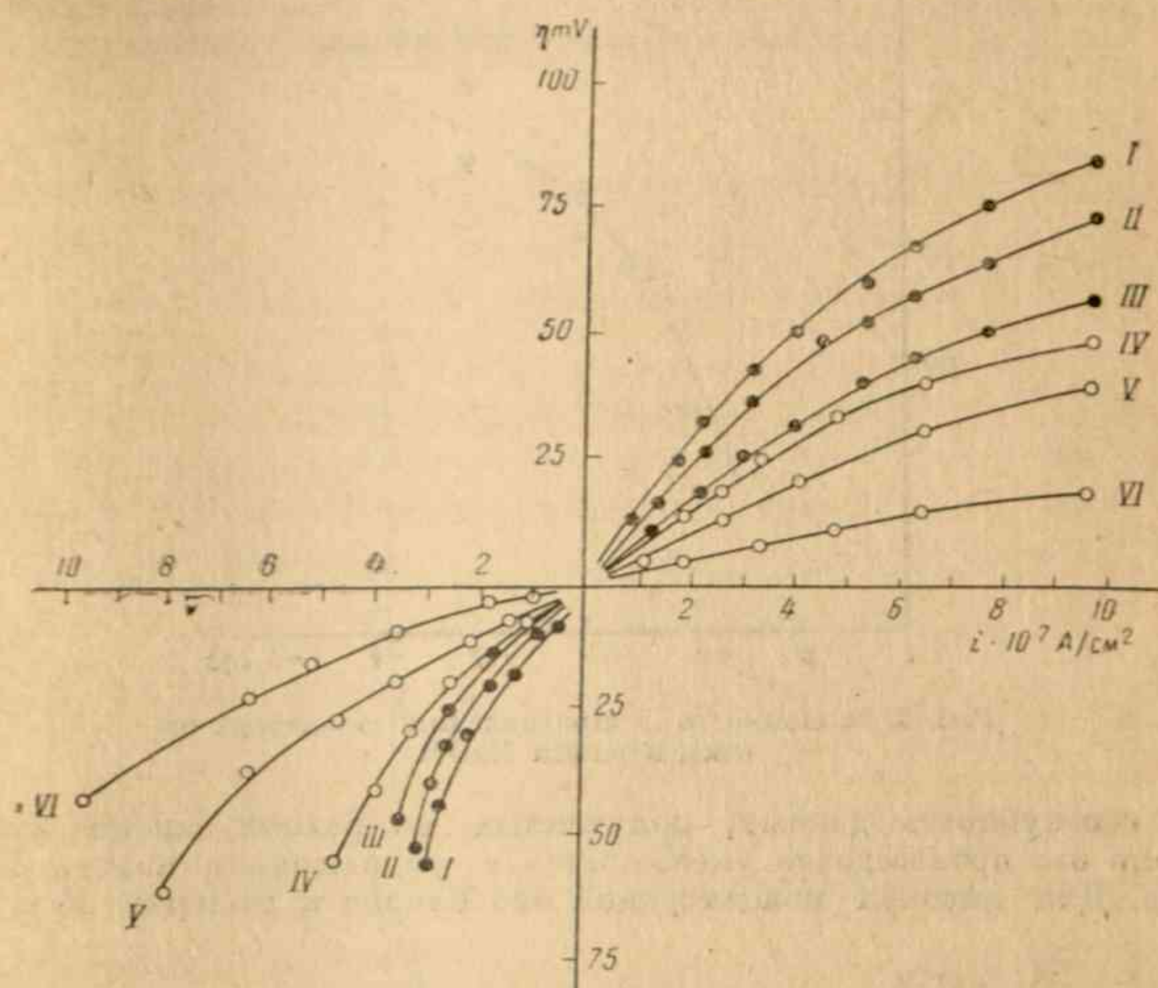
Рис. 5. Зависимость перенапряжения от плотности тока вблизи равновесного потенциала
