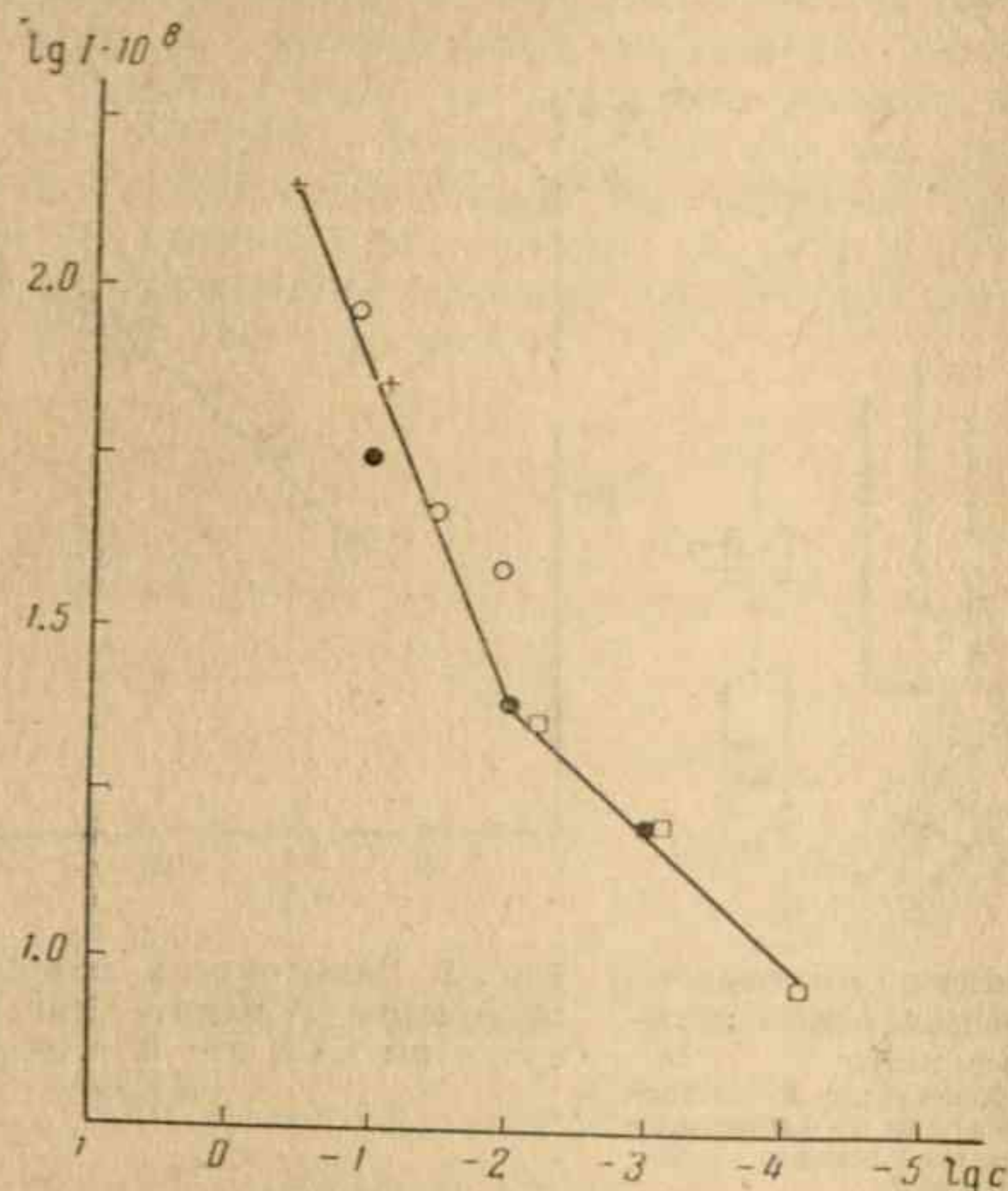
Рис. 4. Зависимость экстраполированного тока обмена от концентрации NaOH
