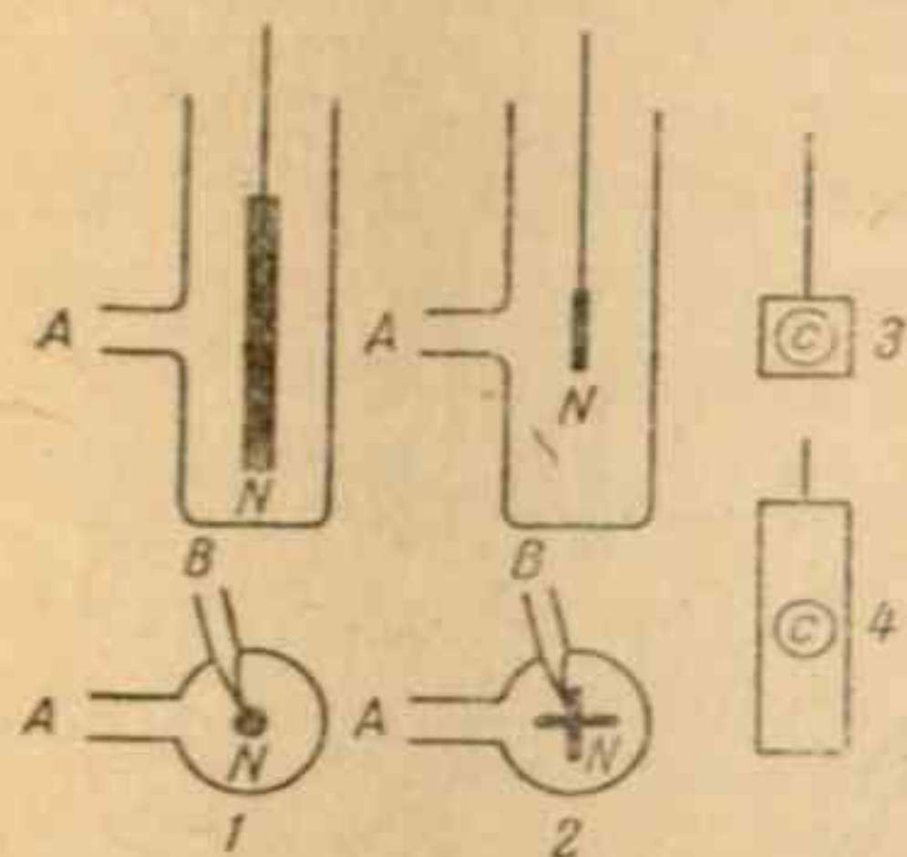
Рис. 2. Положение никелевого электрода N при измерении перенапряжения:
