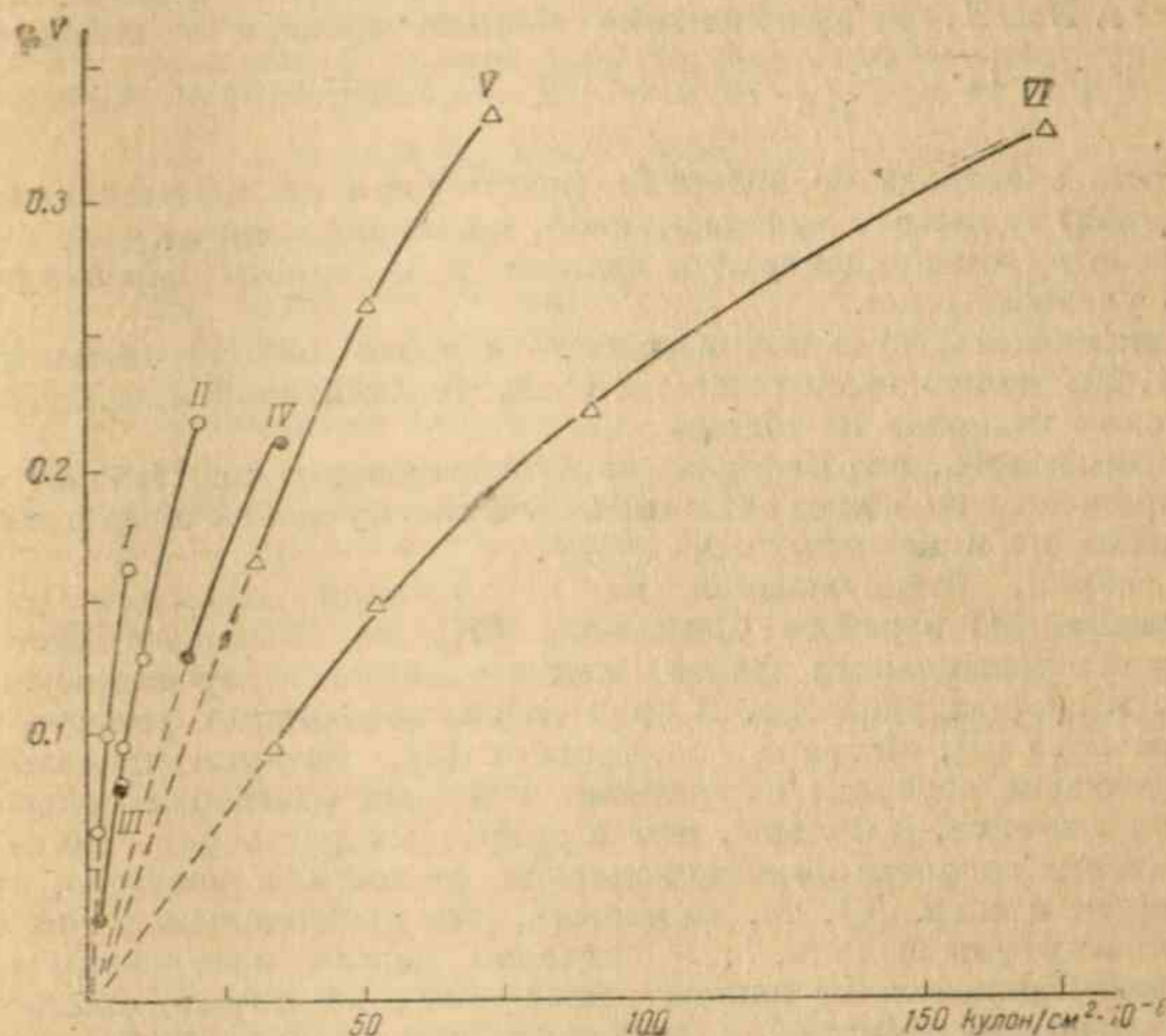
Рис. 10. Зависимость количества электродвижущего вещества от перенапряжения
