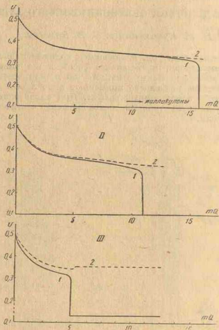
Рис. 2. Изменение потенциалов поляризуемого (сплошные линии) и не поляризуемого (пунктирные линии) контактов в процессе разряда. Сила разрядного тока для кривых:
