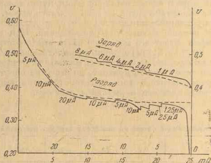
Рис. 3. Изменение потенциалов поляризуемого (сплошные линии) и не поляризуемого (пунктирные линии) контактов в процессе заряда и разряда при изменяющейся силе поляризующего тока. Сила тока (в микроамперах), применявшаяся на каждом участке кривой, записана на чертеже
