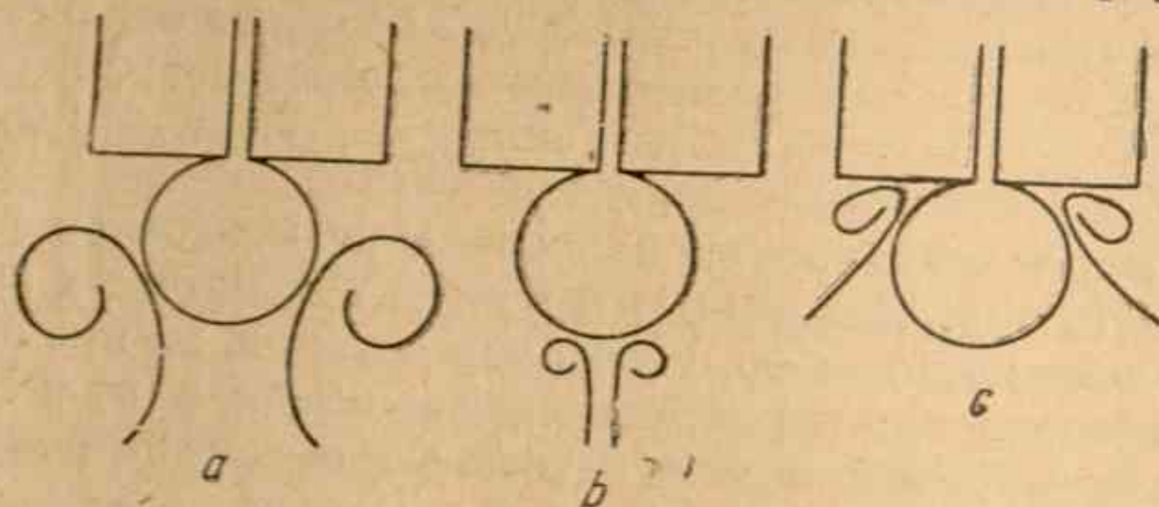
Рис. 2. Разные формы движений раствора возле капли ртути:
