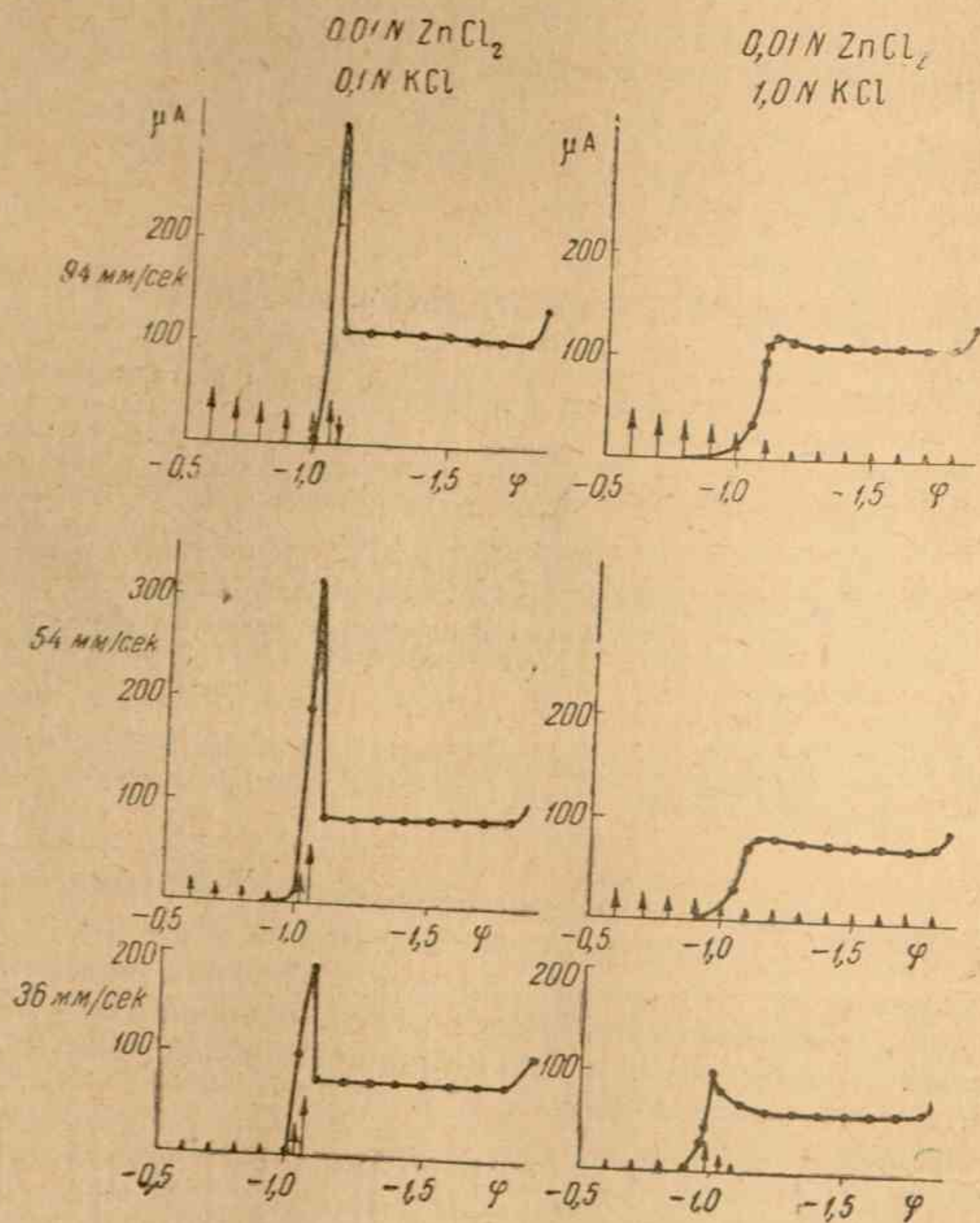
Рис. 7. Поляризационные кривые 0,01 N ZnCl_2 в присутствии 0,1 и 1,0 N KCl при разных скоростях течения ртути в капилляре
