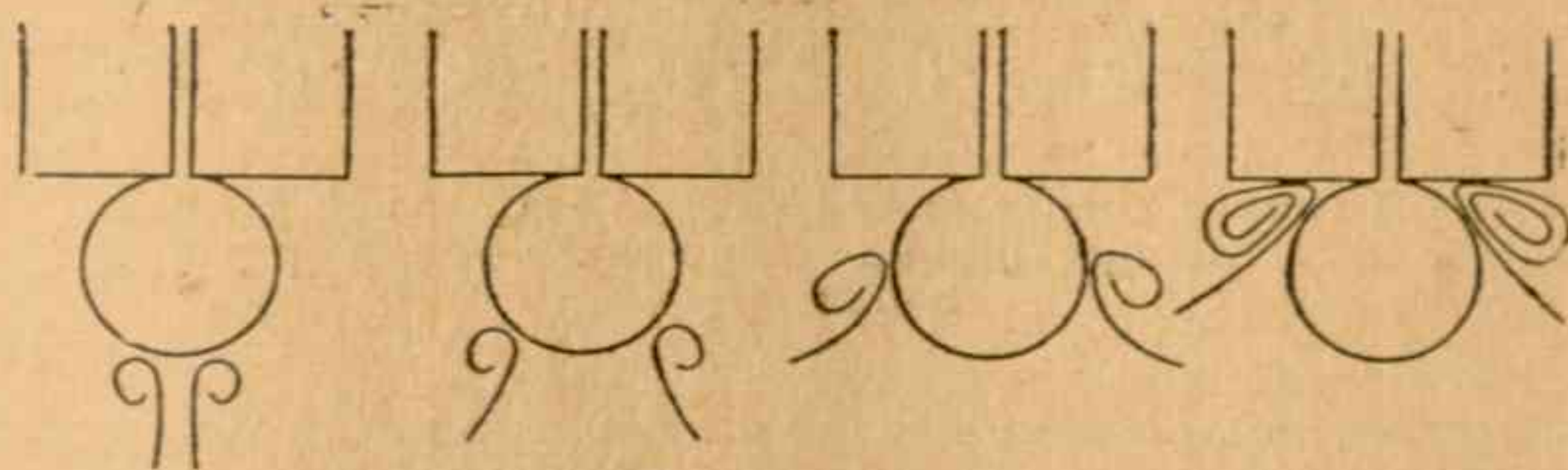
Рис. 6. Перемещение зоны движения поверхности ртути при возникновении отрицательного максимума 1-го рода
