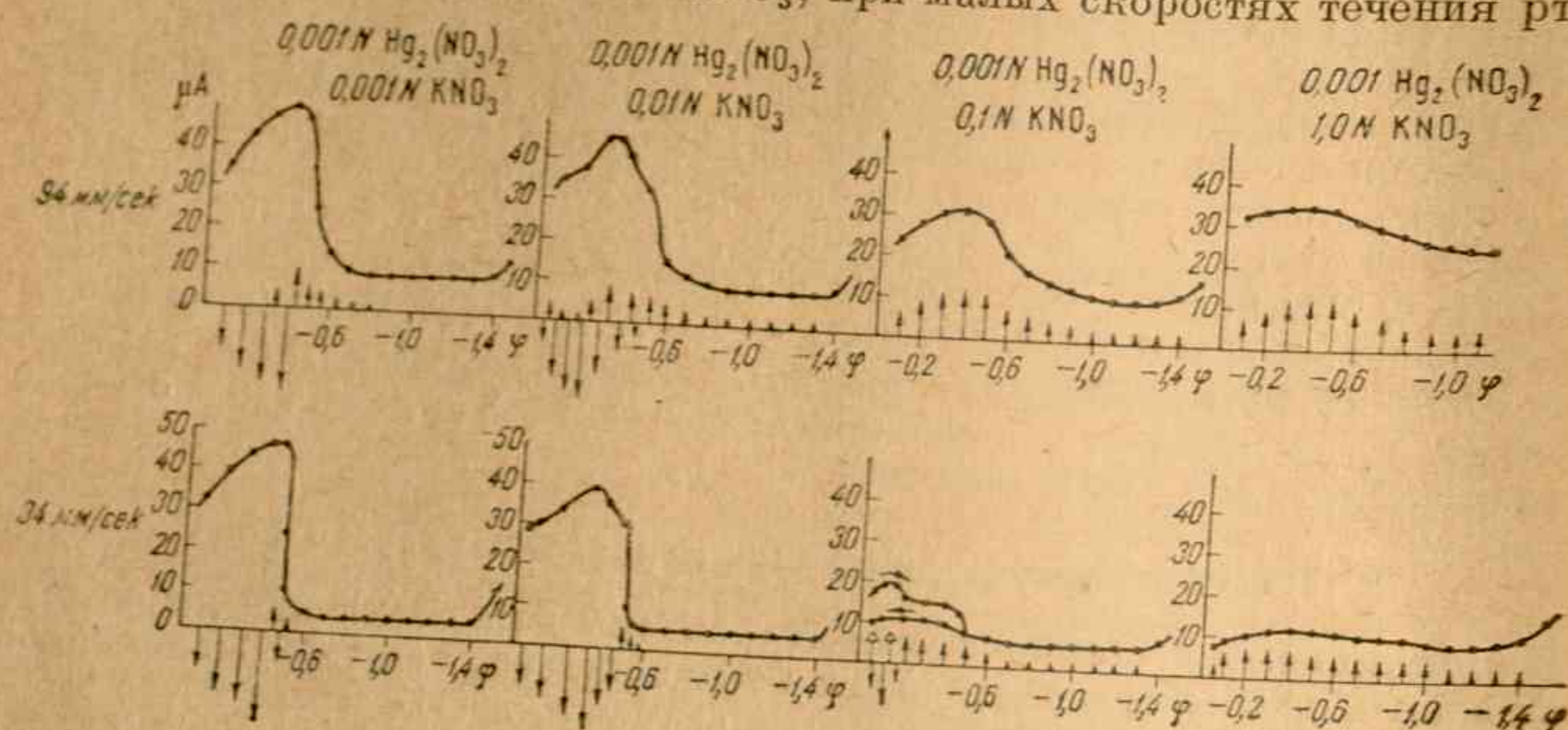
Рис. 4. Кривые i - \varphi 0,001 \text{ N} раствора \text{Hg}_2(\text{NO}_3)_2 и скорости движений раствора возле капли ртути при разных концентрациях \text{KNO}_3 и скоростях течения ртути в капилляре
