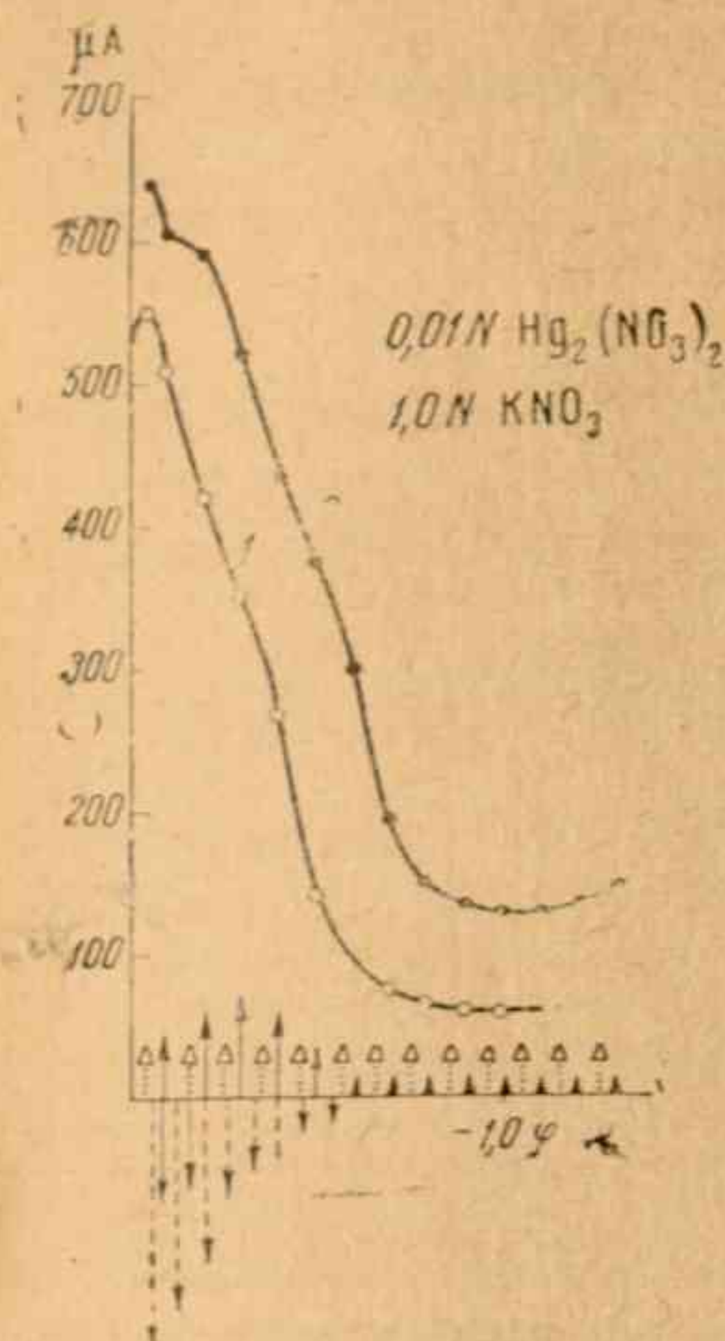
Рис. 5. Инверсия движения 1-го рода в растворе 0,01\text{ N Hg}_2(\text{NO}_3)_2 + 1,0\text{ N KNO}_3
