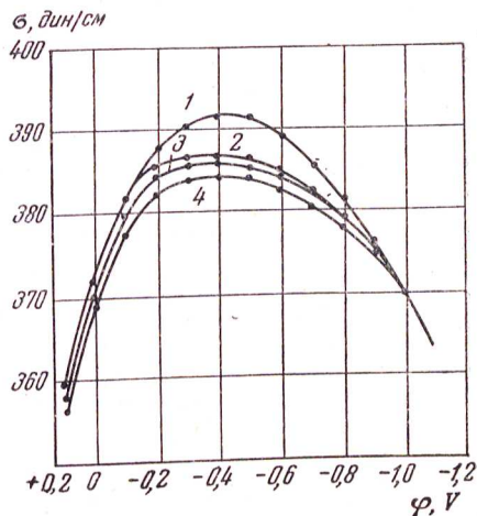
Рис. 2. Электрокапиллярные кривые растворов пятичленных циклических углеводородов в метиловом спирте: 1 — метилового спирта + 0,2 моль/л \text{NH}_4\text{NO}_3 ; 2 — метилциклопентана 1,0 моль/л; 3 — метилциклопентена-2, 1,0 моль/л; 4 — метилциклопентена-1, 1,0 моль/л
