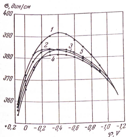
Рис. 1. Электрокапиллярные кривые растворов шестичленных циклических углеводородов в метиловом спирте: 1 — метилового спирта + 0,2 моль/л \text{NH}_4\text{NO}_3 ; 2 — циклогексана 1,0 моль/л; 3 — циклогексана 1,0 моль/л; 4 — циклогексана-1,3 1,0 моль/л; 5 — бензола 1,0 моль/л
