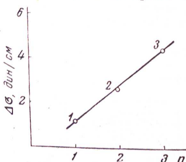
Рис. 3. Кривая, характеризующая зависимость адсорбционной активности от числа двойных связей в молекуле: 1 — циклогексен; 2 — циклогексадиен-1,3; 3 — бензол
