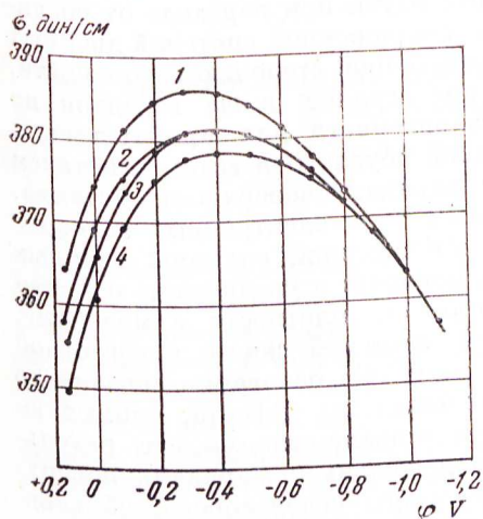
Рис. 4. Электрокапиллярные кривые растворов гидроантрацена в метиловом спирте: 1 — этиловый спирт + 0,2 моль/л \text{NH}_4\text{NO}_3 ; 2 — октагидроантрацена 0,002 моль/л; 3 — тетрагидроантрацена 0,002 моль/л; 4 — антрацена 0,002 моль/л
