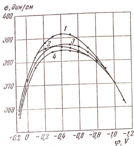
Рис. 5. Электрокапиллярные кривые растворов непредельных алифатических углеводородов в метиловом спирте: 1 — метиловый спирт + 0,2 моль/л \text{NH}_4\text{NO}_3 ; 2 — n -гептана и гептена 1,0 моль/л; 3 — гексадиена-1,5 1,0 моль/л; 4 — гексадиен-2 41,0 моль/л
