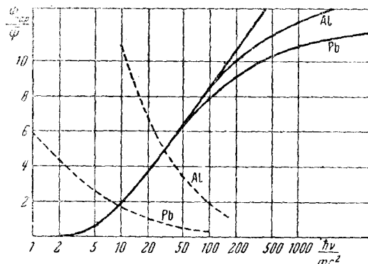
Рис. 3. Эффективный поперечник для образования пар \psi_{\text{пар}} как функция частоты падающих \gamma -квантов в логарифмической шкале. Единицы \bar{\psi} = \frac{Z^2 r_0^2}{137} . Пунктирные кривые представляют эффективный поперечник для комптон-эффекта в тех же единицах. Левая верхняя кривая показывает ход \psi_{\text{пар}} без учета экранирования
