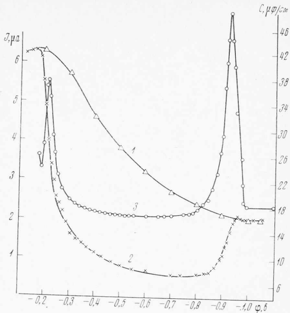
Рис. 4. Сопоставление C , \Phi - и I , \Phi -кривых при концентрации адмантанол-1 6 \cdot 10^{-5} мол/л: 1 — C , \Phi -кривая в 1 M \text{Na}_2\text{SO}_4 ; 2 — то же в 1 M \text{Na}_2\text{SO}_4 + адмантанол-1; 3 — I , \Phi -кривая в 10^{-3} N \text{AgNO}_3 + 1 M \text{Na}_2\text{SO}_4 + адмантанол-1
