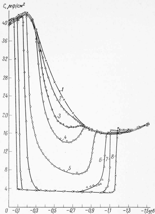
Рис. 2. Зависимость дифференциальной емкости от потенциала в 1 M Na_2SO_4 с добавками адамантанола-1: 1—0; 2— 2 \cdot 10^{-5} M ; 3— 2,5 \cdot 10^{-5} ; 4— 3 \cdot 10^{-5} ; 5— 6 \cdot 10^{-5} ; 6— 1 \cdot 10^{-4} ; 7— 1,8 \cdot 10^{-4} ; 8— 3 \cdot 10^{-4} M
