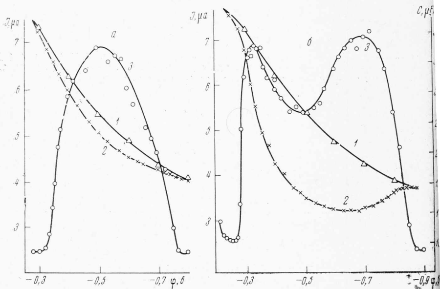
Рис. 3. Сопоставление C, \phi - и I, \phi -кривых при различных концентрациях п.а.в. (2 \cdot 10^{-5} , 6— 3 \cdot 10^{-5} мол/л адамантанола-1): 1— C, \phi -кривая в 1 M Na_2SO_4 ; 2—то же в 1 M Na_2SO_4 + адамантанол-1; 3— I, \phi -кривая в 1 M Na_2SO_4 + 10^{-3} N AgNO_3 + адамантанол-1
