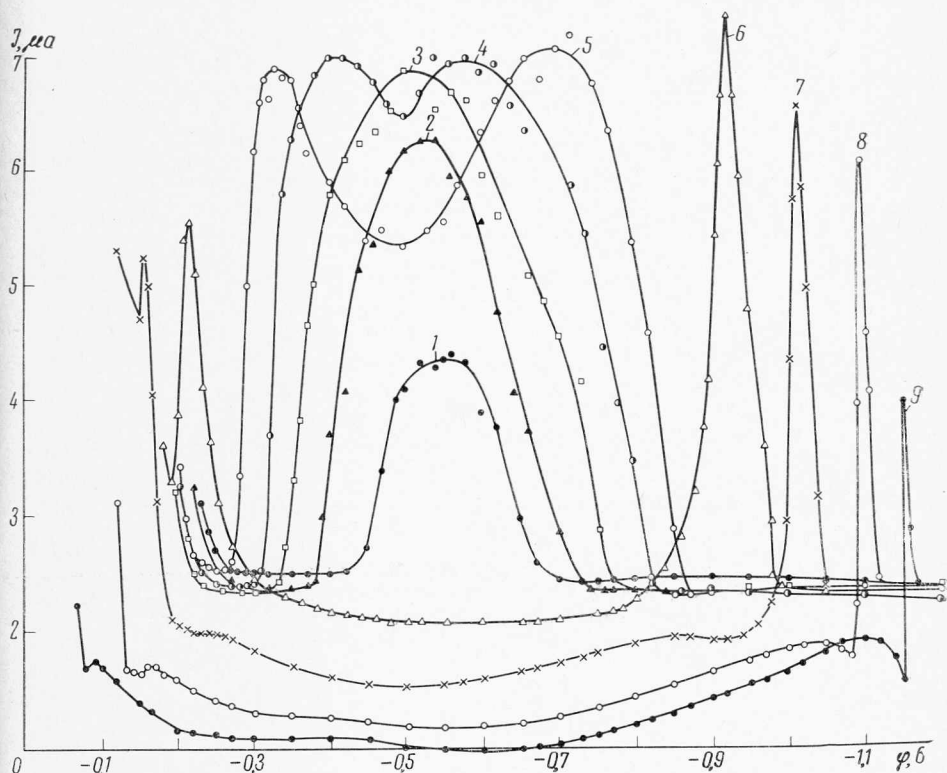
Рис. 1. Зависимость тока от потенциала при восстановлении 10^{-3} N \text{ AgNO}_3 + 1 M \text{ Na}_2\text{SO}_4 с добавками адамантанола-1: 1 — 1,5 \cdot 10^{-5} M ; 2 — 1,7 \cdot 10^{-5} ; 3 — 2 \cdot 10^{-5} ; 4 — 2,5 \cdot 10^{-5} ; 5 — 3 \cdot 10^{-5} ; 6 — 6 \cdot 10^{-5} ; 7 — 1 \cdot 10^{-4} ; 8 — 1,8 \cdot 10^{-4} ; 9 — 3 \cdot 10^{-4} мол/л
