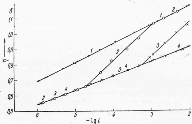
Рис. 1. Перенапряжение в 1 N HCl в присутствии дифениламина. 1 — 1N HCl; 2 — 1N HCl + 1,34 \cdot 10^{-5} М дифениламин; 3 — 1N HCl + 4,3 \cdot 10^{-4} М дифениламин; 4 — 1N HCl + 1,34 \cdot 10^{-3} М дифениламин
