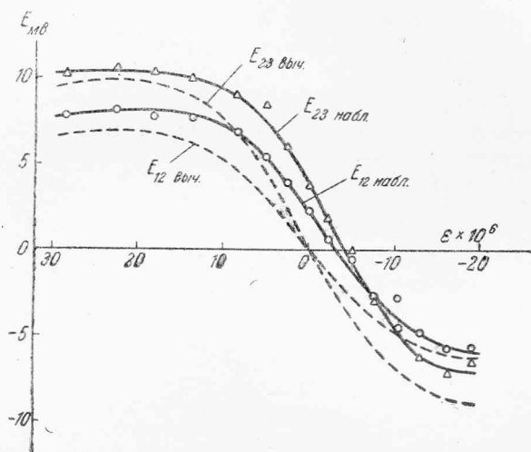
Рис. 2. Зависимость потенциала падающих капель E_{12} и E_{23} от плотности зарядов \epsilon в 1 N растворе KBr в глицерине!
