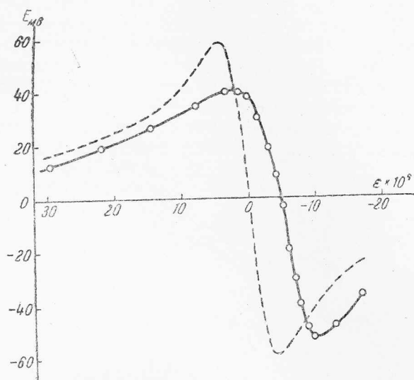
Рис. 4. Зависимость потенциала падающих капель E_{12} от плотности зарядов \epsilon в 0,015 N растворе KBr в глицерине
