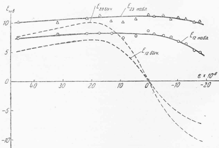
Рис. 5. Зависимость потенциала падающих капель E_{12} и E_{23} от плотности зарядов \epsilon в 1 N растворе KBr в глицерине при неполном удалении кислорода;
