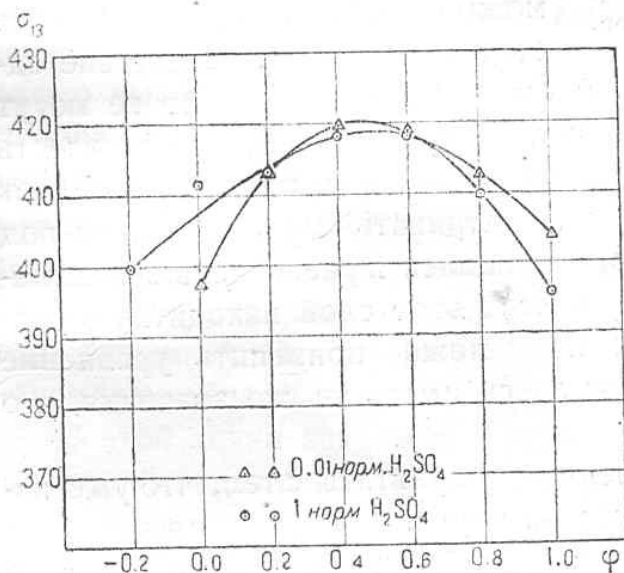
Рис. 7. Пограничное натяжение ртуть—пузырек в растворах неорганических электролитов.
