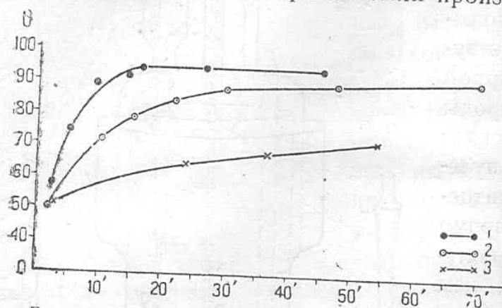
Рис. 3. Изменение краевого угла со временем. 1 диаметр пузырька 0,2 мм. 2 " " 0,4 мм. 3 " " 1,7 мм.
