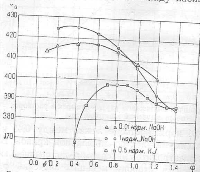
Рис. 8. Пограничное натяжение ртути—пузырек в растворах неорганических электролитов.
