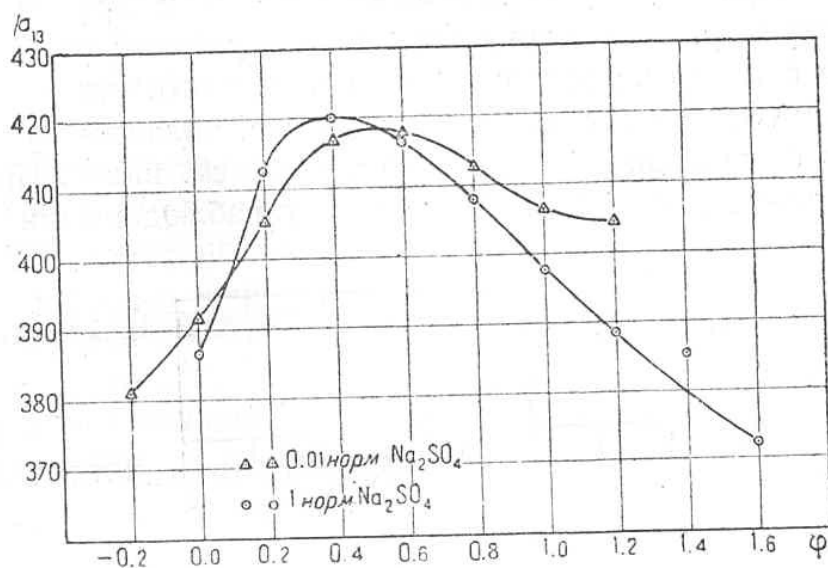
Рис. 6. Пограничное натяжение ртуть—пузырек в растворах неорганических электролитов.
