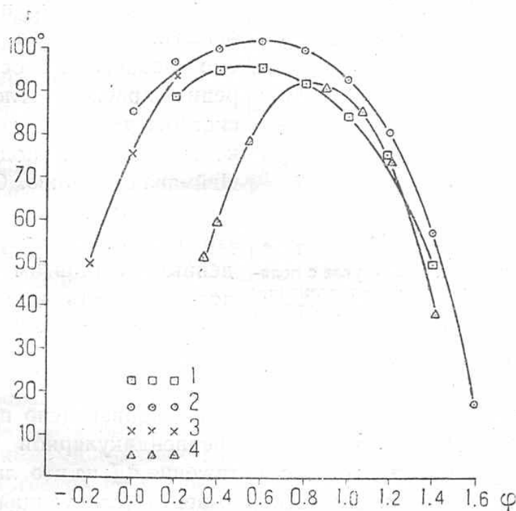
Рис. 4. Кривые изменения краевого угла с поляризацией для водных растворов электролитов.
