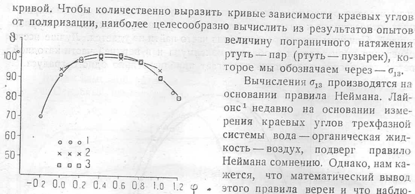
Рис. 5. Кривые изменения краевого угла с поляризацией для водных растворов электролитов. 1—0,01 норм. Na 2 SO 4 , 2—0,01 норм. H 2 SO 4 , 3—0,01 норм. NaOH
