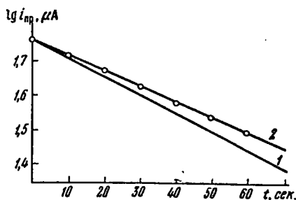
Рис. 5. Микрокулонометрирование \text{BrO}_3^- в кислой среде; состав раствора: 10^{-3}M \text{ KBrO}_3 + 10^{-1}N \text{ H}_2\text{SO}_4 + 1,0N \text{ K}_2\text{SO}_4 + 0,01\% желатин. Сплошные линии — рассчитанные по уравнению Джильберта и Райделя [12]: 1 — n=5 ; 2 — n=6 ; кружки — экспериментальные точки
