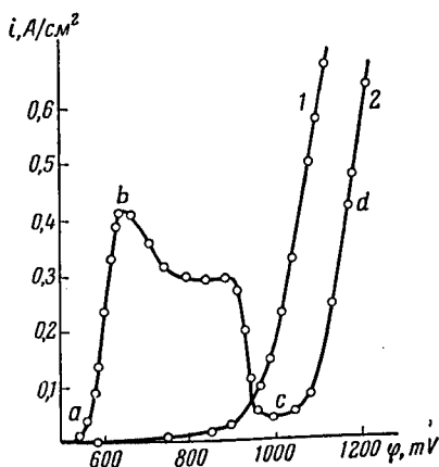
Рис. 1. Поляризационные кривые, снятые в хромовой кислоте на хромовом катоде. Кривая 1 снята в отсутствие серной кислоты; 2 — снята в присутствии 5 г/л \text{H}_2\text{SO}_4
