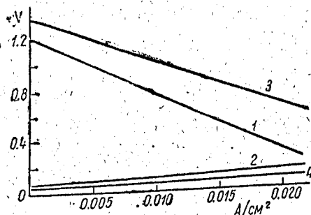
Рис. 6. Влияние образования перекиси водорода на потенциалы электродов в элементе при t = -15^\circ .
