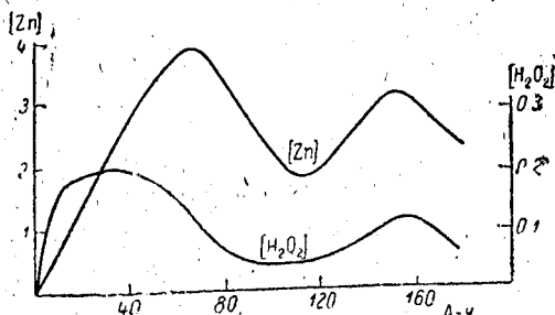
Рис. 2. Кривые изменения концентрации перекиси водорода, а также цинката в электролите при t = 15^\circ в электролите из 35% КОН.
