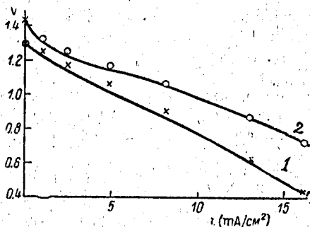
Рис. 9. Влияние катализатора на поляризацию угольного электрода ВД при t = 0^\circ .
