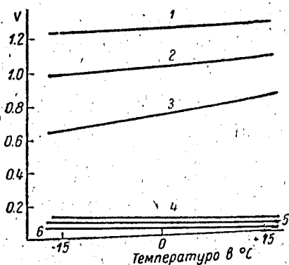
Рис. 8. Кривые зависимости потенциала угольного и цинкового электродов от температуры в отсутствии образования перекиси водорода для плотности тока: 1 и 6 — 0.004, 2 и 5 — 0.01 и 3 и 4 — 0.02 \text{A}/\text{cm}^2 .
