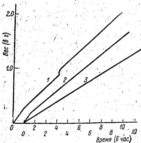
Рис. 1. Кривые увеличения веса работающего элемента со временем.
