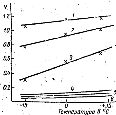
Рис. 7. Кривые зависимости потенциала угольного и цинкового электродов от температуры в случае образования перекиси водорода в элементе для плотности тока: 1 и 6 — 0.004, 2 и 5 — 0.01 и 3 и 4 — 0.02, \text{A}/\text{cm}^2 .
