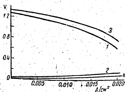
Рис. 5. Влияние образования перекиси водорода на потенциалы электродов в элементе при t = 15^\circ .
