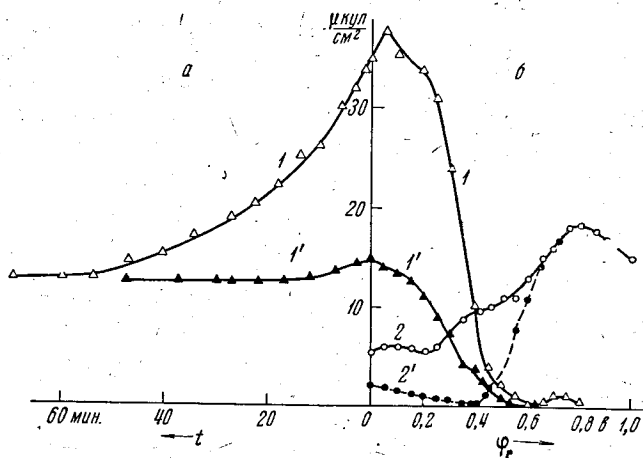
Рис. 3. а — зависимость количества оставшихся на поверхности адсорбированных катионов \text{Zn}^{2+} от времени обмена. 1 — в отсутствие и 1' — в присутствии хемосорбированного метанола при \phi_r = 0 в растворе 10^{-2} \text{ N H}_2\text{SO}_4 + 3 \cdot 10^{-3} \text{ N ZnSO}_4 ; б — зависимость адсорбции катионов \text{Zn}^{2+} (1, 1') и анионов \text{SO}_4^{2-} (2, 2') от потенциала в том же растворе; 1, 2' — на поверхности, свободной от метанола, 1', 2' — в присутствии хемосорбированного метанола
