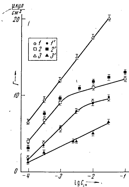
Рис. 2. Зависимость величин адсорбции катионов от их концентрации в растворе при φ r = 0. 1 — Na + (pH 3); 2 — Cs + (pH 3) и 3 — Zn 2+ (pH 0) в отсутствие хемосорбированного метанола. 1', 2', 3' — то же в присутствии хемосорбированного метанола
