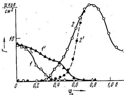
Рис. 1. Зависимость адсорбции ионов от потенциала электрода: 10 -3 N H 2 SO 4 + 3·10 -3 N Na 2 SO 4 . Na + (1) и SO 4 2- (2) на поверхности, свободной от метанола; Na + (1') и SO 4 2- (2') — в присутствии хемосорбированного метанола
