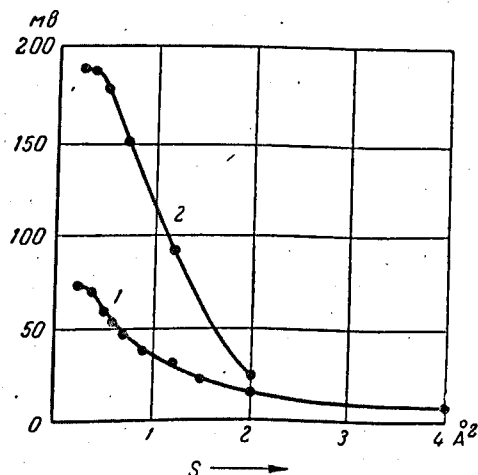
Рис. 2. Зависимость поверхностного потенциала от площади на молекулу для пленки фенантрена. 1 — на растворе 3 N KCl, 2 — на растворе 4 N \text{CaCl}_2
