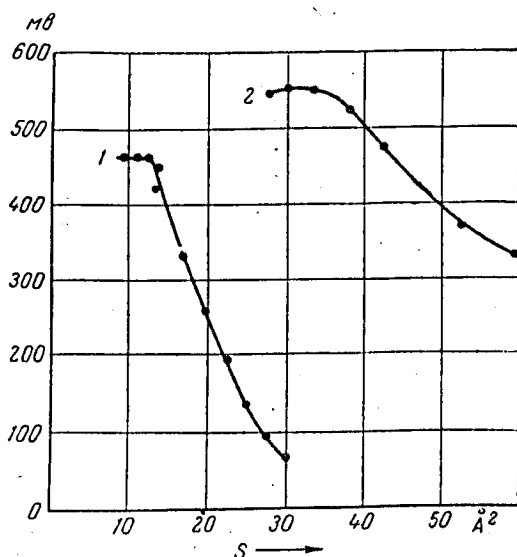
Рис. 4. Зависимость поверхностного потенциала от площади на молекулу для пленки тетрацена. 1 — на воде, 2 — на 8 N \text{CaCl}_2
