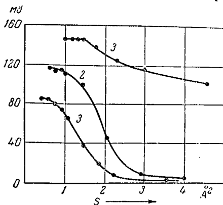
Рис. 3. Зависимость поверхностного потенциала от площади на молекулу для пленки антрацена. 1 — на воде, 2 — на 3 N KCl, 3 — на 8 N \text{CaCl}_2
