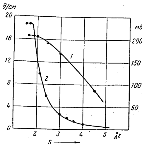
Рис. 1. Зависимость поверхностного потенциала (1) и двухмерного давления (2), от площади на молекулу для пленки фенантрена на растворе 8 N \text{CaCl}_2
