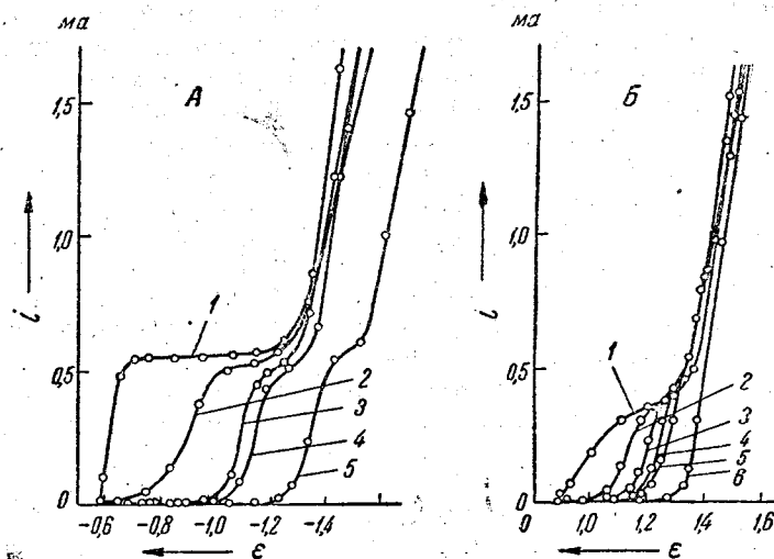
Рис. 2. Влияние добавок на полярографические волны кадмия и хрома. А — электролит 0,06 N CdSO 4 , 1 N H 2 SO 4 ; 1 — чистый раствор, 2 — м-крезол (0,005 М/л); 3 — ментол (насыщенный); 4 — ксиленол-1-3-4 (насыщенный); 5 — камфора (насыщенный). Б — электролит 0,05 N Cr 2 (SO 4 ) 3 , 1 N H 2 SO 4 ; 1 — чистый раствор; 2 — м-крезол (0,005 М/л); 3 — октиловый спирт (насыщенный); 4 — ксиленол-1-3-4 (насыщенный); 5 — эвгенол (насыщенный); 6 — камфора (насыщенный)
