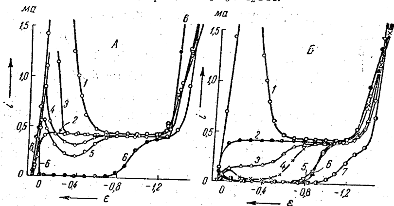
Рис. 1. Полярограммы выделения меди из чистого CuSO_4 (кривая 1) и из растворов с добавками поверхностно-активных веществ. Состав раствора: 0,05 N CuSO_4 и 1 N H_2SO_4 . А — в раствор введены желатина (кривая 2), 0,005 M ксидина (3), 0,005 и 0,01 M бензилового спирта (4 и 5) и камфора до насыщения (6). Б — в раствор добавлено 0,05 г/л \beta -нафтола (3), 0,01\% желатины (2), 0,05 M бензилового спирта (4), карвакрола (5), ксиленола до насыщения (6) и трибензиламина 0,005 M (7).
